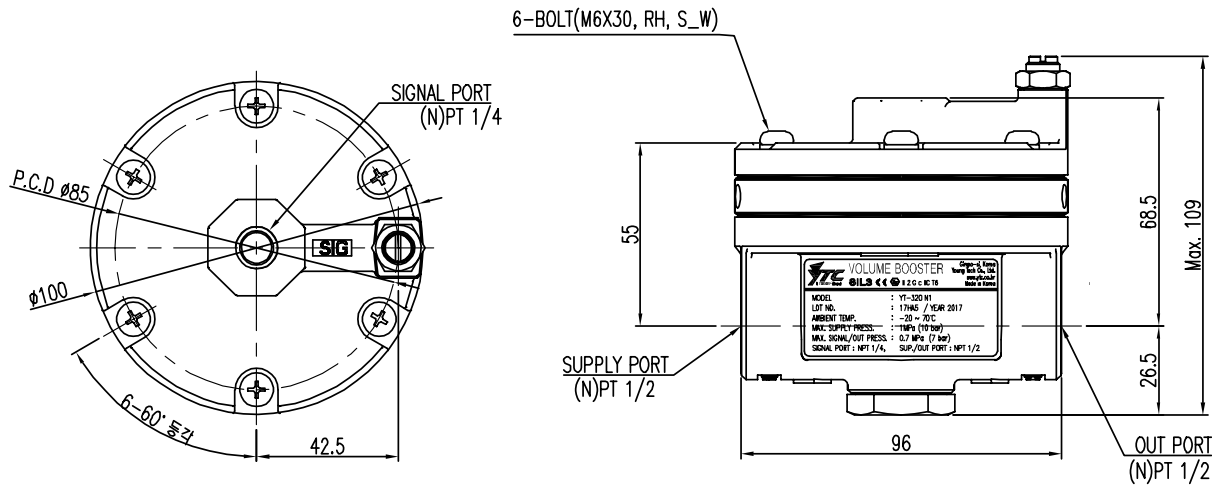
Fig. 2-7: YT-320 / 325 dimension
